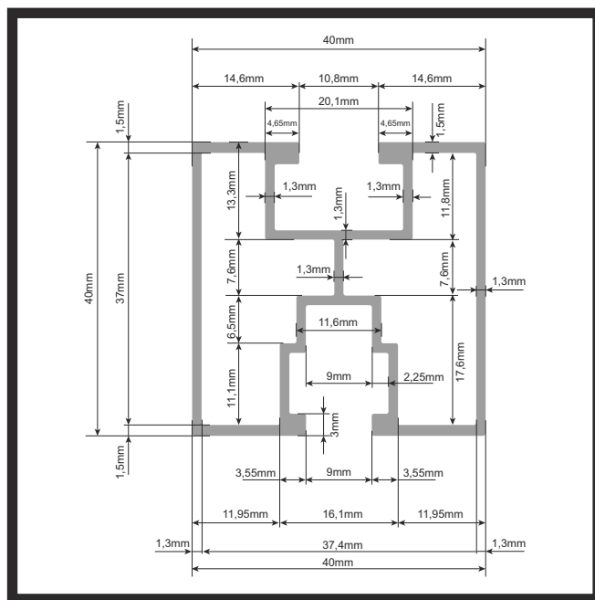
PV PROFILE ID: SP2T0,797P1600 Дължина - 6м. / Цена: 8,00 лв./м.
