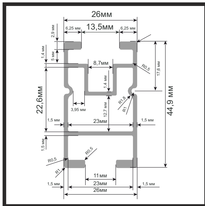
PV PROFILE ID: SP15T0,797P1716 Дължина - 6м. / Цена: 8,00 лв./м.
